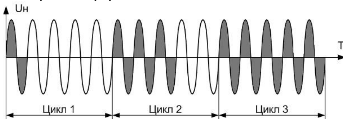
Рисунок 3.6 Выходное напряжение при регулировании методом пропуска периодов
