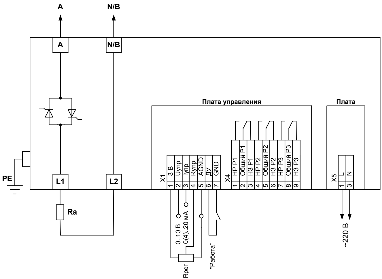
Рисунок А1 Схема подключения
