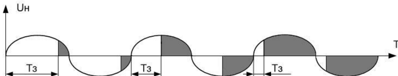
Рисунок 3.4 Выходное напряжение при фазовом способе регулирования
