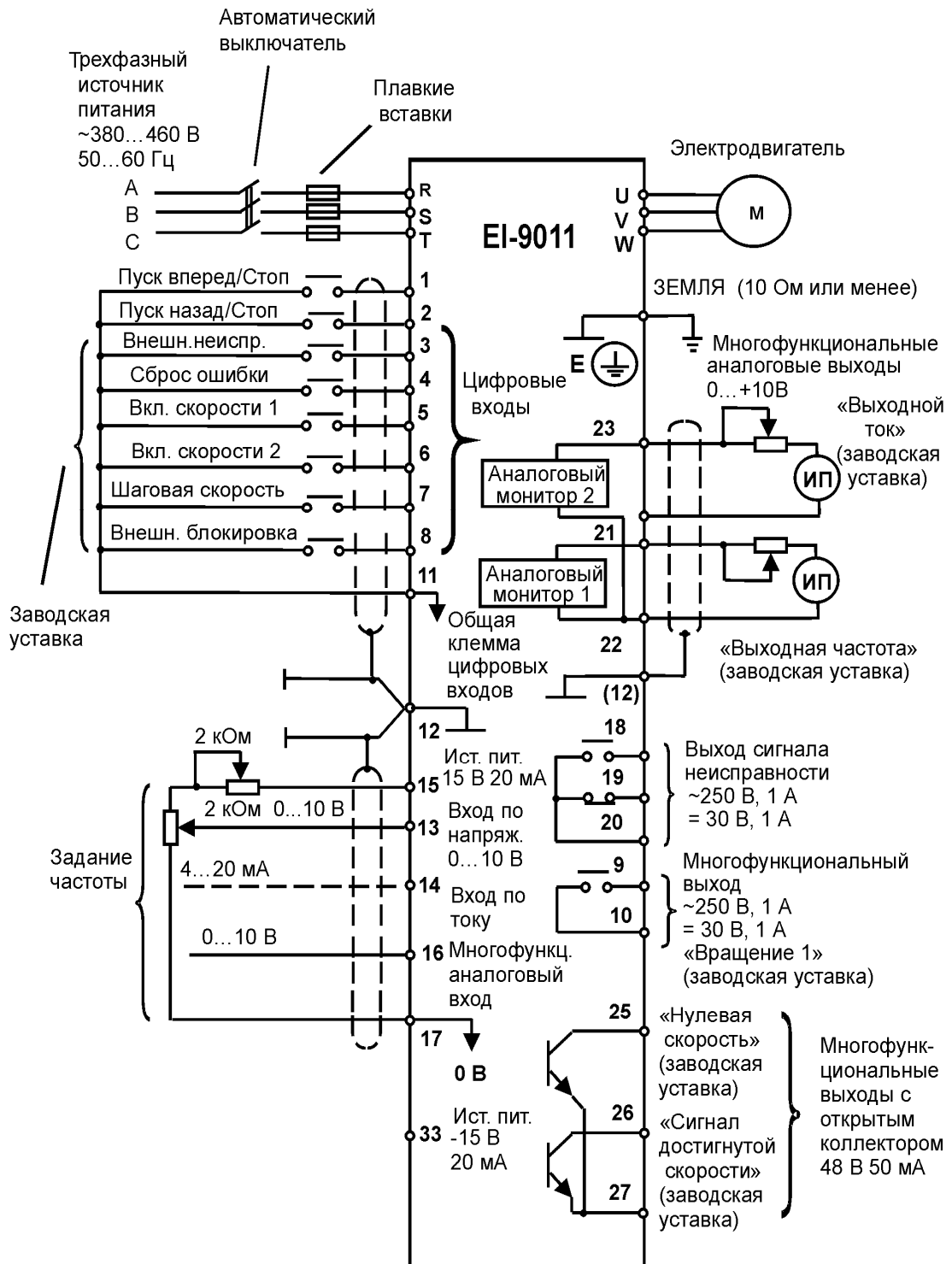
Рис. 4. Схема подсоединения
