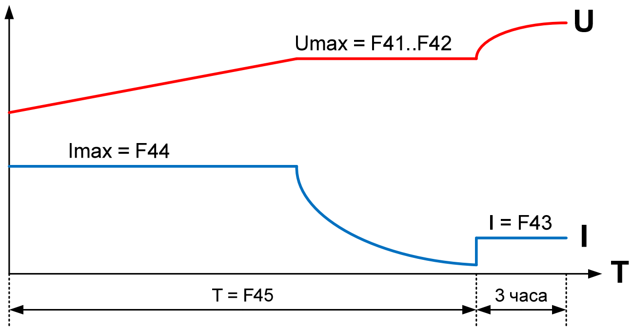
Рисунок 3.2 Диаграмма напряжений и токов в режиме уравнительного заряда
