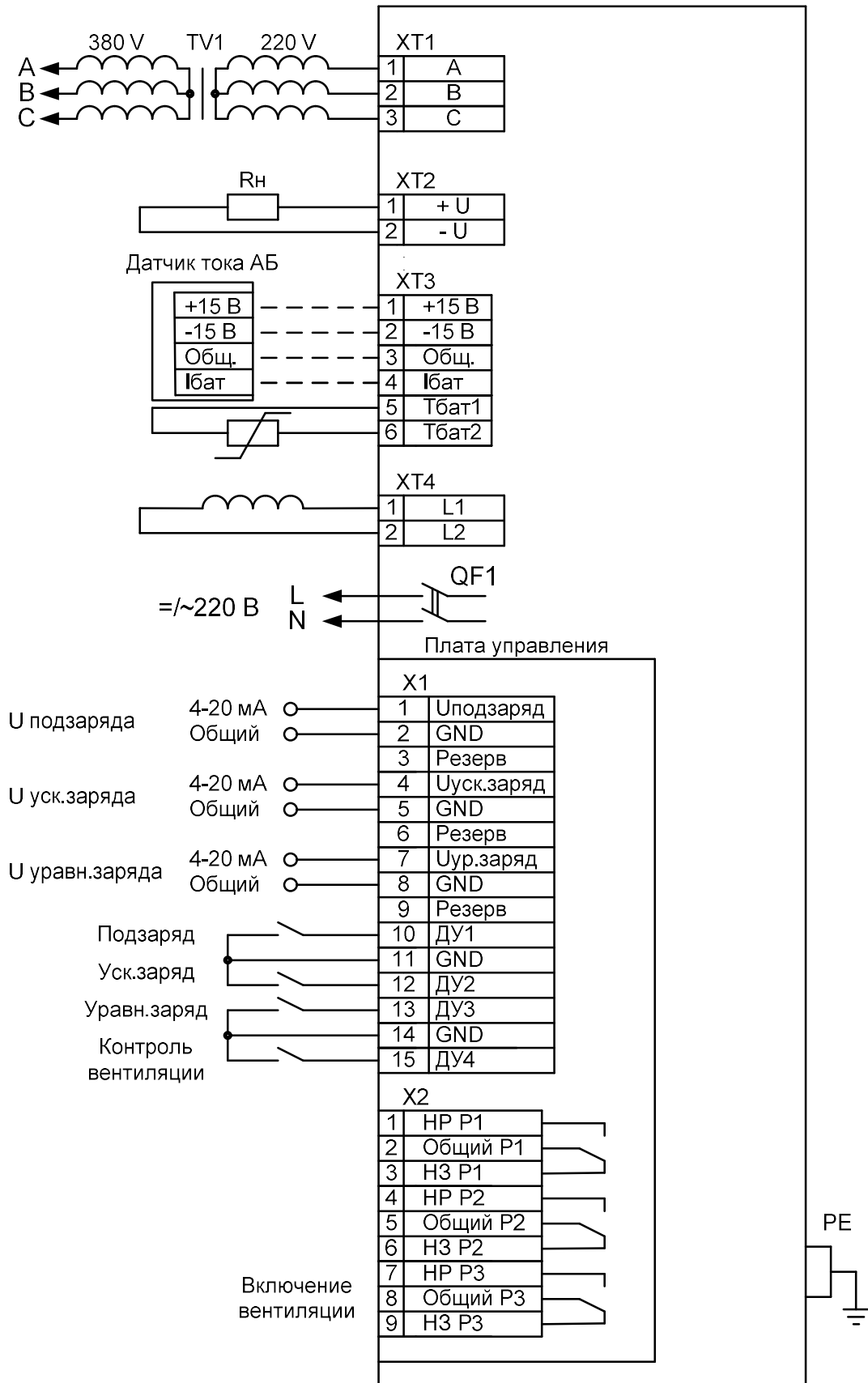
Рисунок А1 Схема подключения
