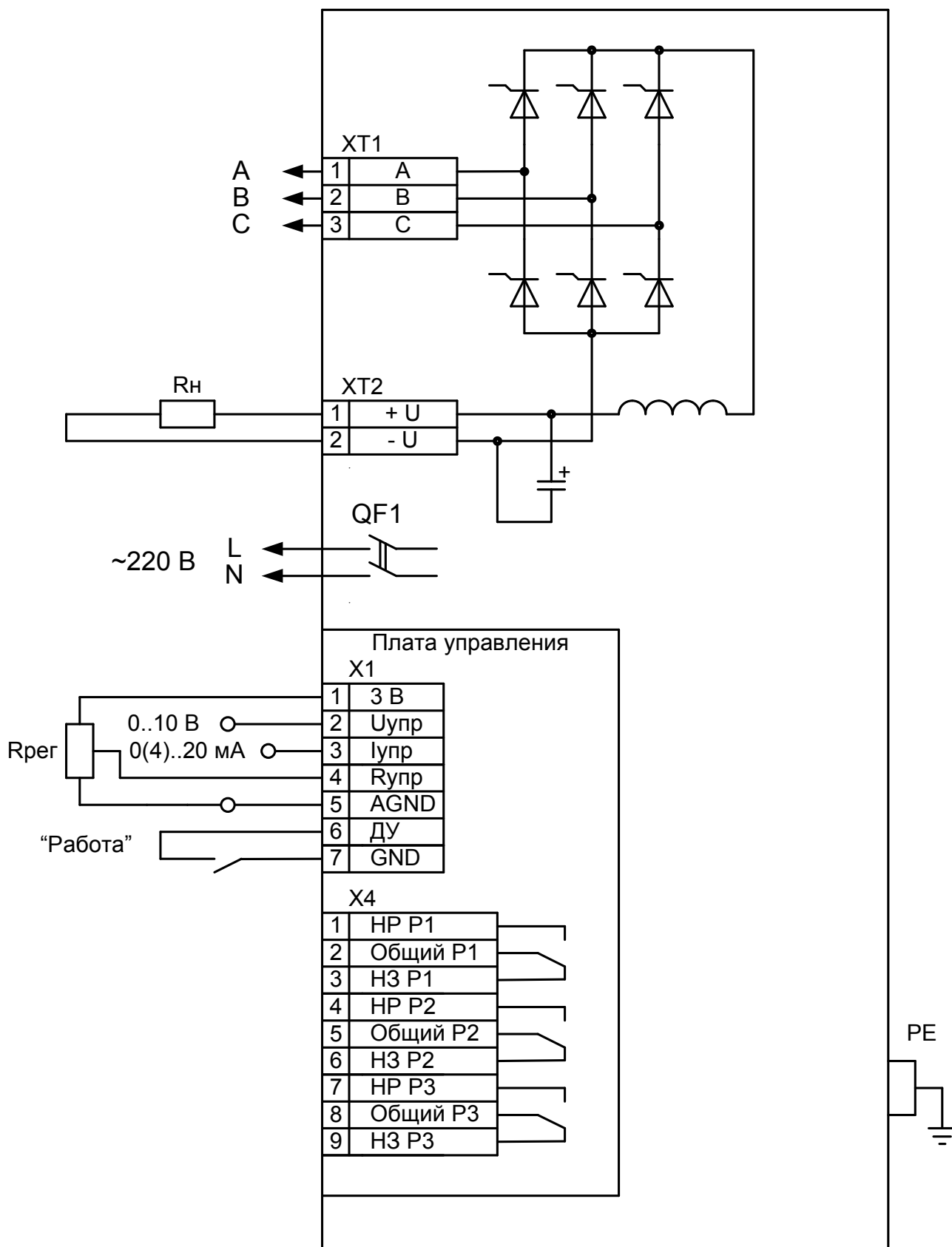
Рисунок А1 Схема подключения
