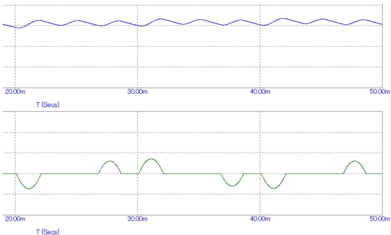
Рисунок 3.3 Выходное напряжение выпрямителя(вверху) и ток в фазе(внизу) со сглаживающим дросселем фильтром
