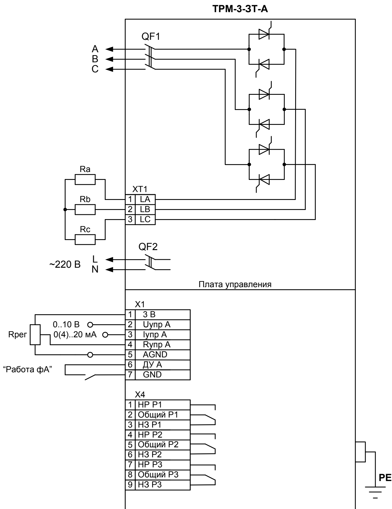
Рисунок А1 Схема подключения нагрузки – “звезда”
