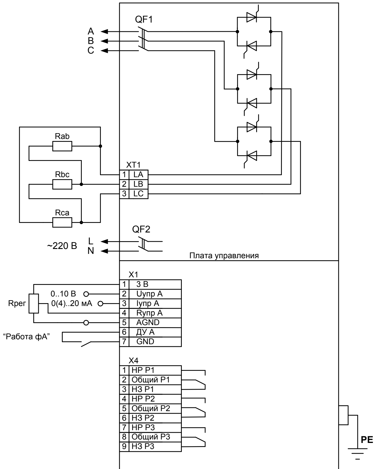
Рисунок А2 Схема подключения нагрузки – "треугольник"
