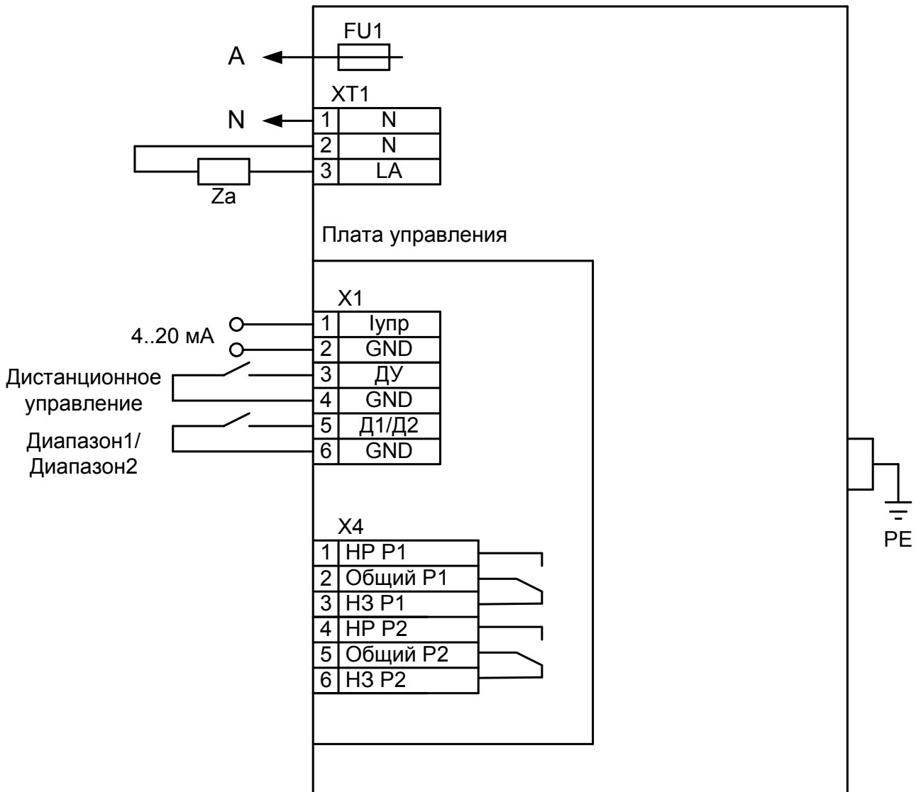
Рисунок А1 Схема внешних проводок устройства
