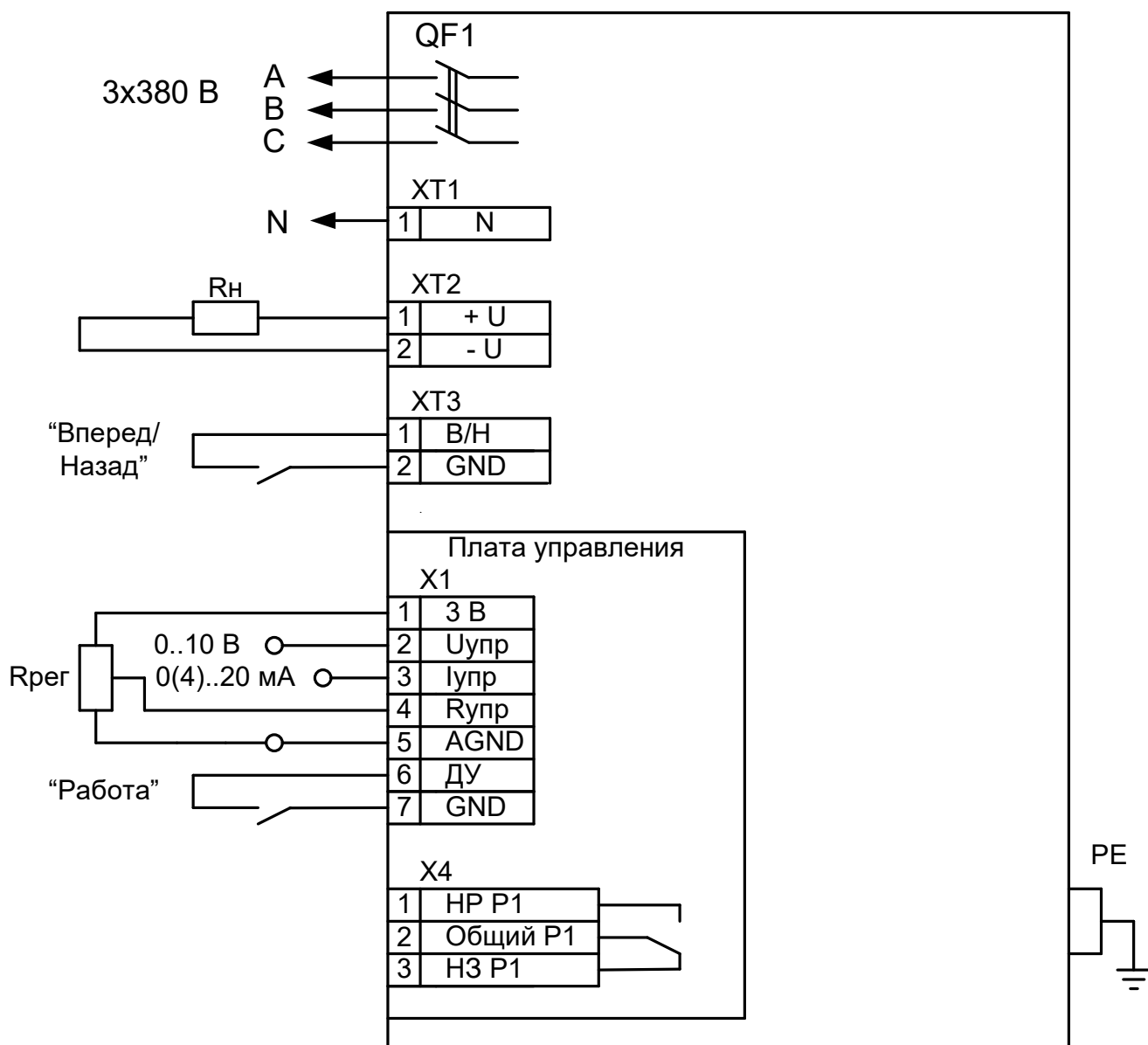
Рисунок А1 Схема подключения РБП-Р-576-62, питание – трехфазное с нулевым проводом
