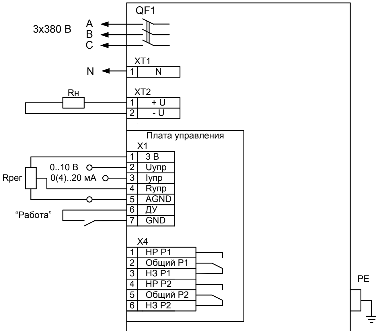
Рисунок А3 Схема подключения РБП-96-125, РБП-96-187, РБП-96-250, питание – трехфазное с нулевым проводом
