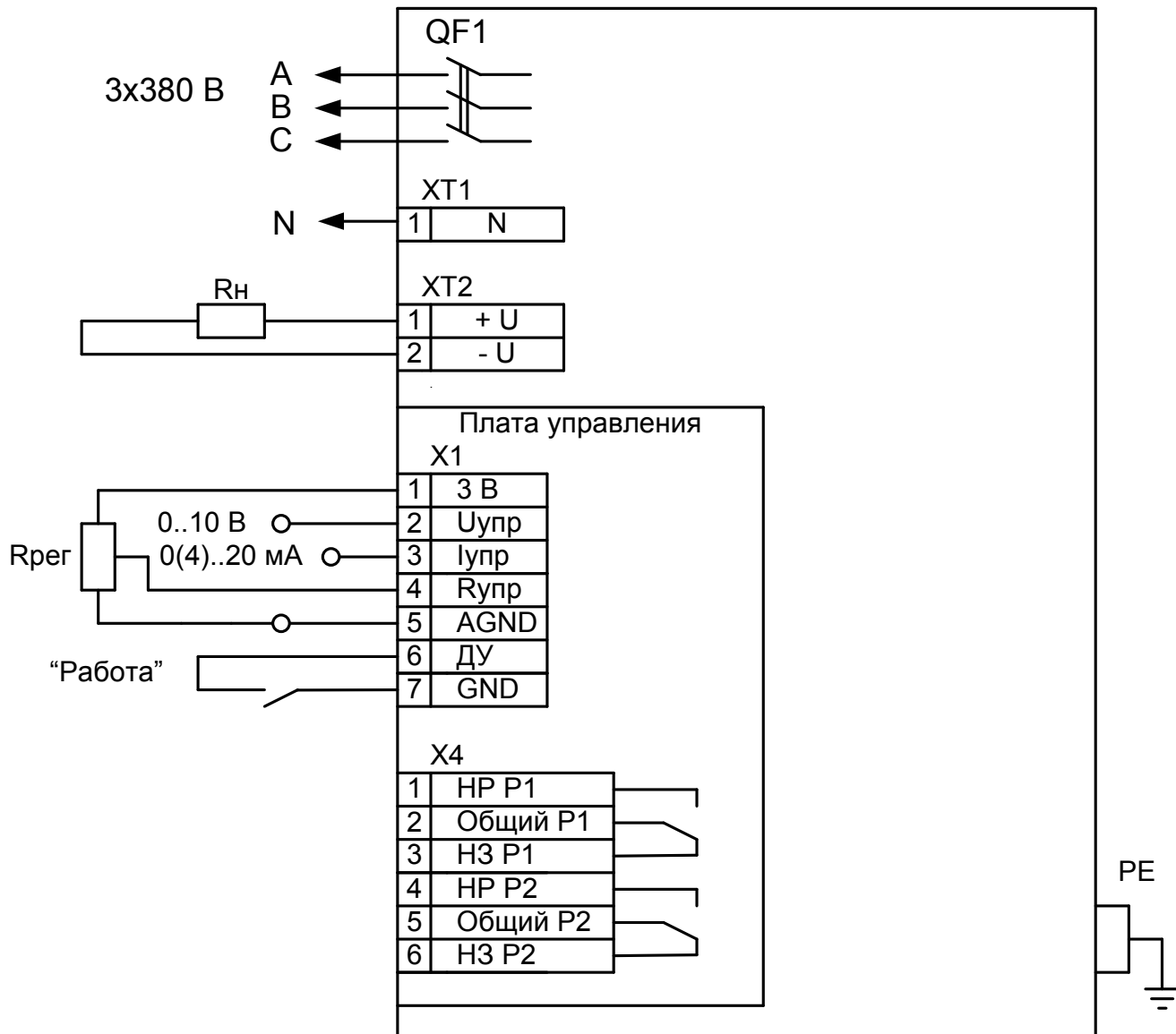
Рисунок А1 Схема подключения РБП-72-125, РБП-72-250, питание – трехфазное с нулевым проводом
