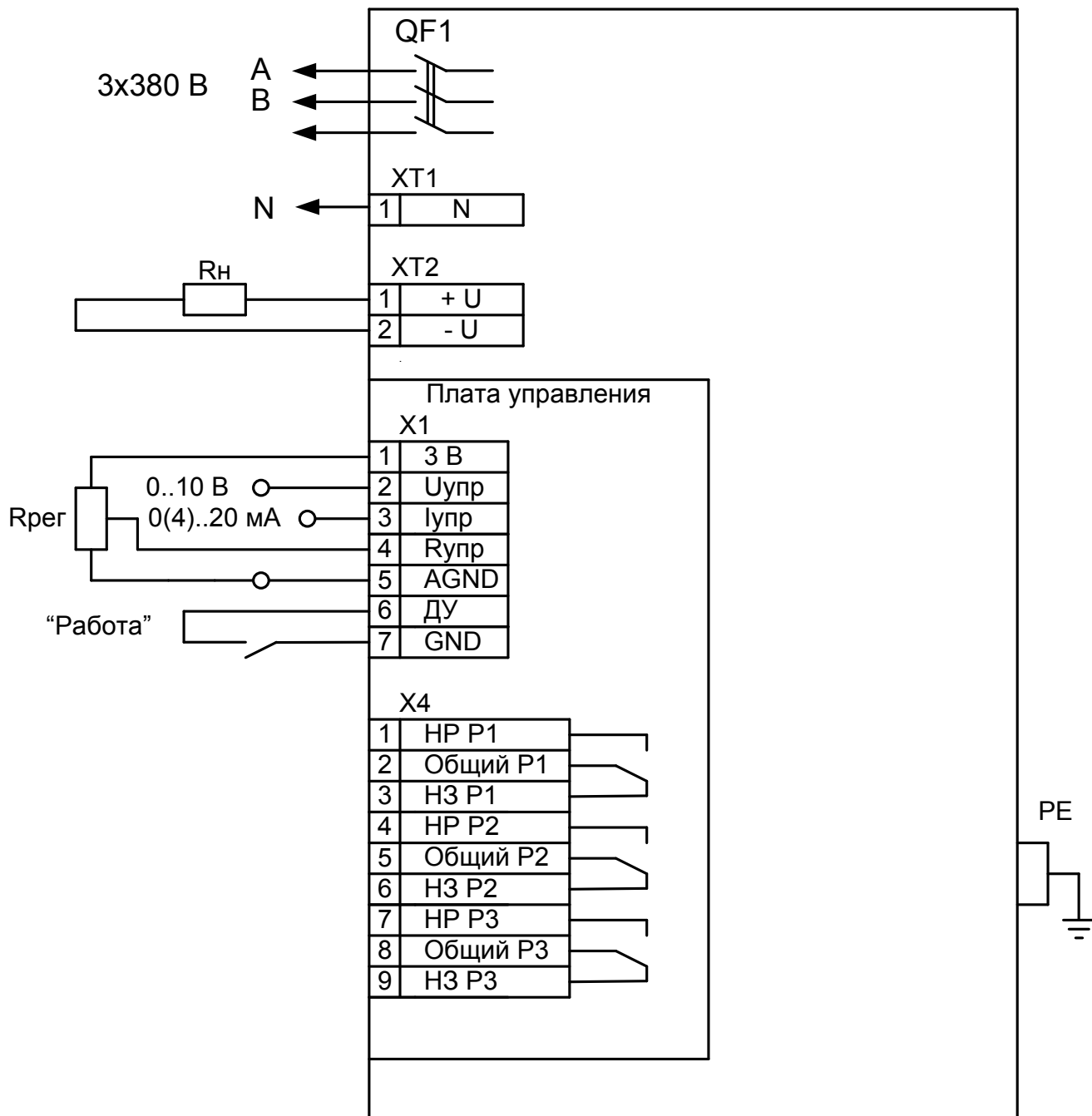
Рисунок А3 Схема подключения РБП-36-200, РБП-36-400, РБП-36-600, питание – трехфазное с нулевым проводом
