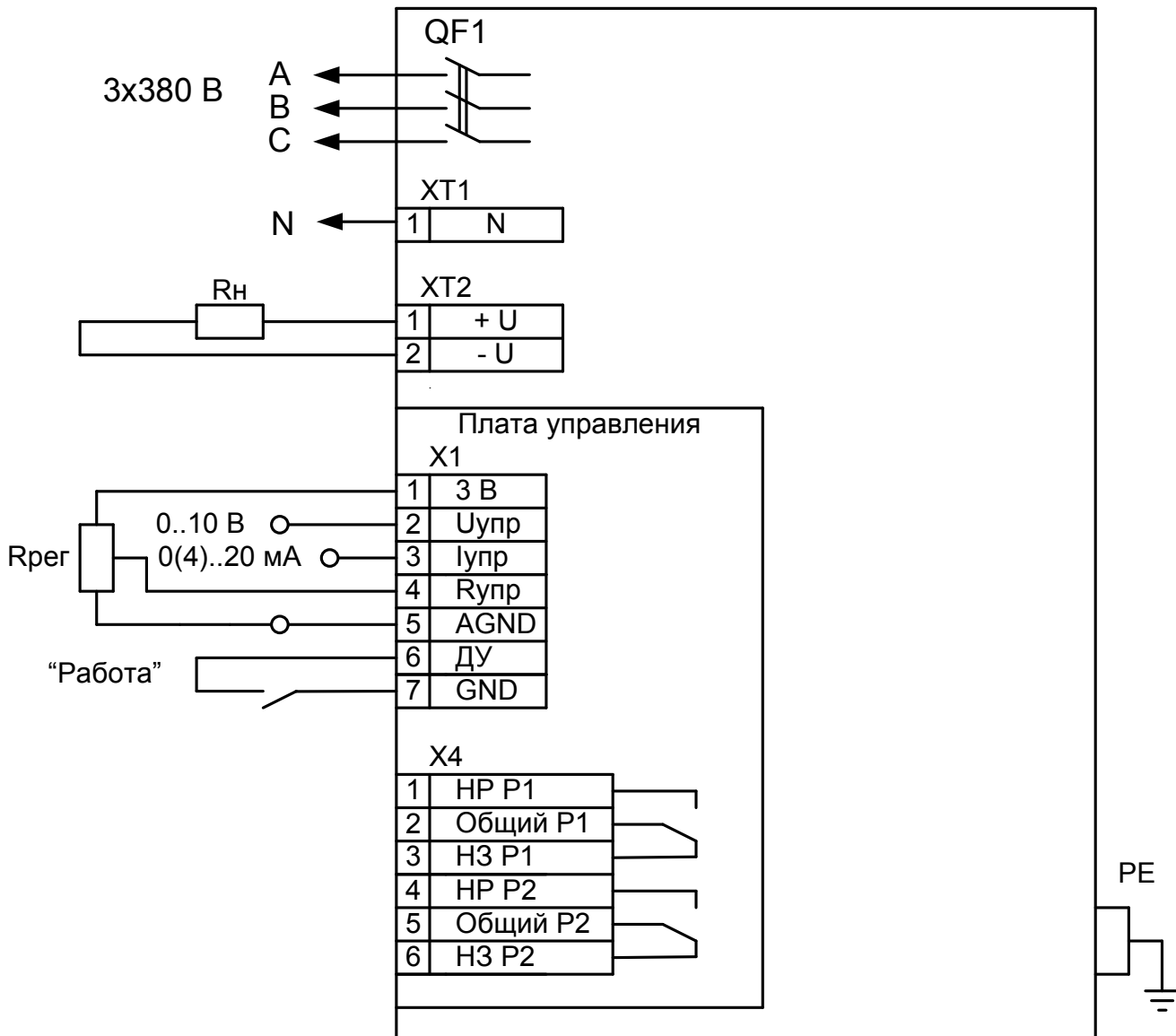
Рисунок А1 Схема подключения РБП-288-62, питание – трехфазное с нулевым проводом
