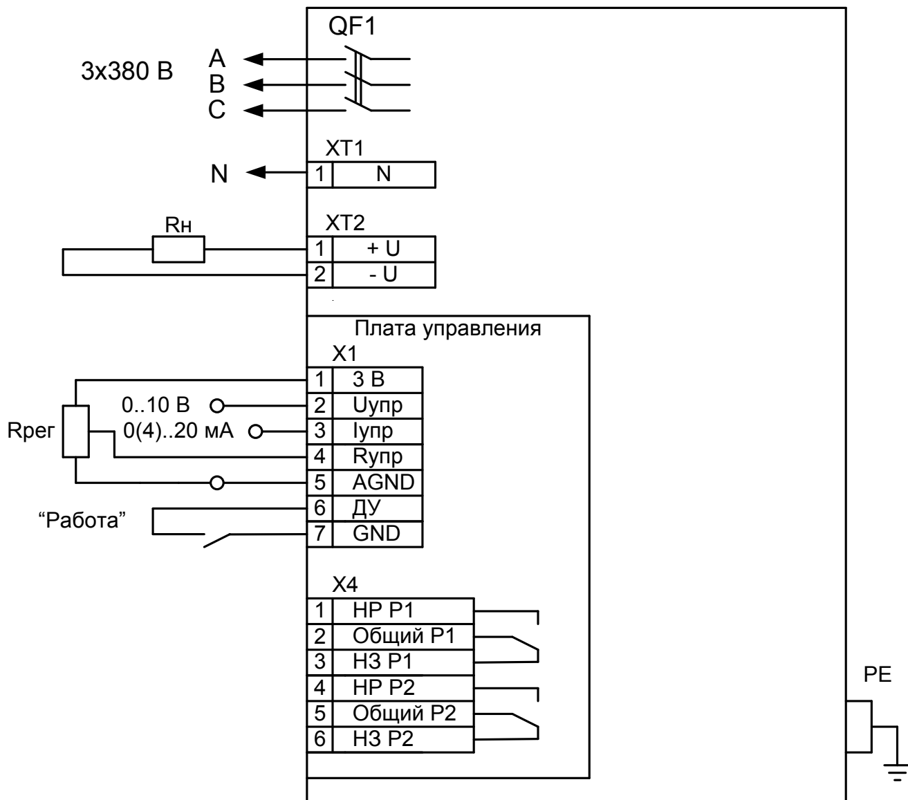
Рисунок А1 Схема подключения РБП-192-62, РБП-192-125, питание – трехфазное с нулевым проводом
