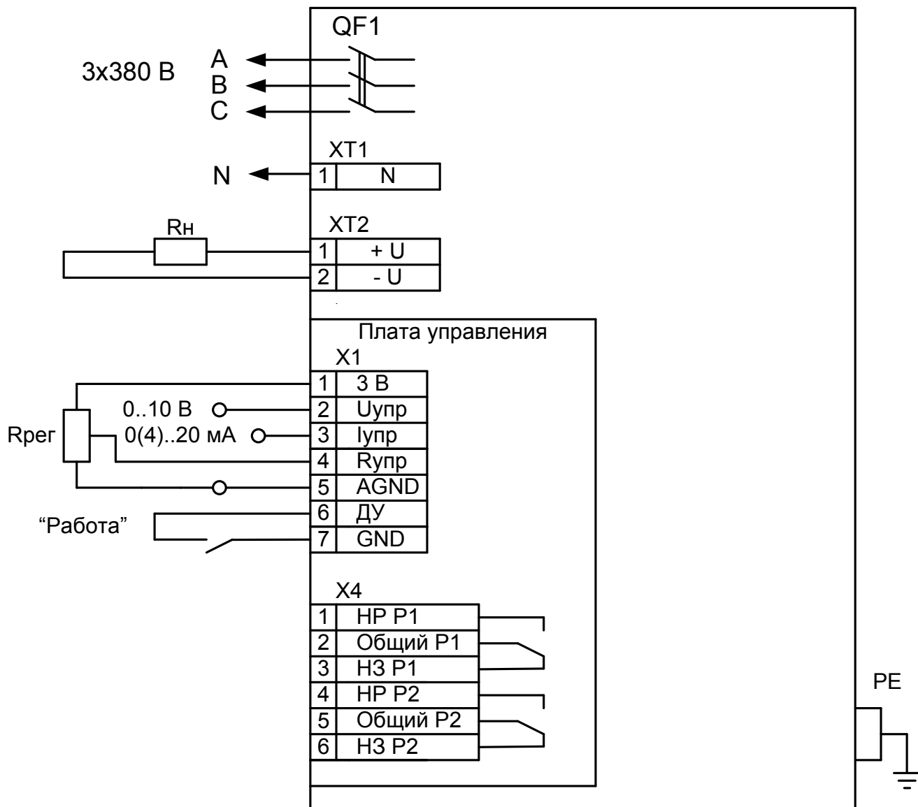
Рисунок А1 Схема подключения РБП-144-62, РБП-144-125, РБП-144-187 питание – трехфазное с нулевым проводом
