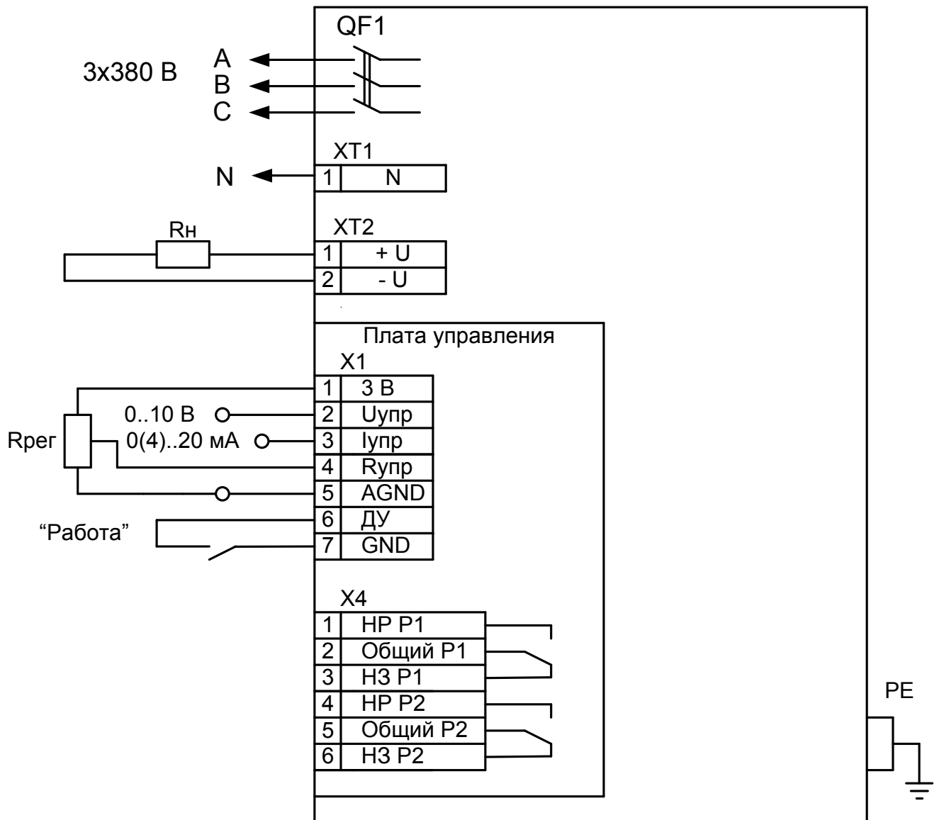
Рисунок А3 Схема подключения РБП-12-600, РБП-12-800, РБП-12-1000, питание – трехфазное с нулевым проводом
